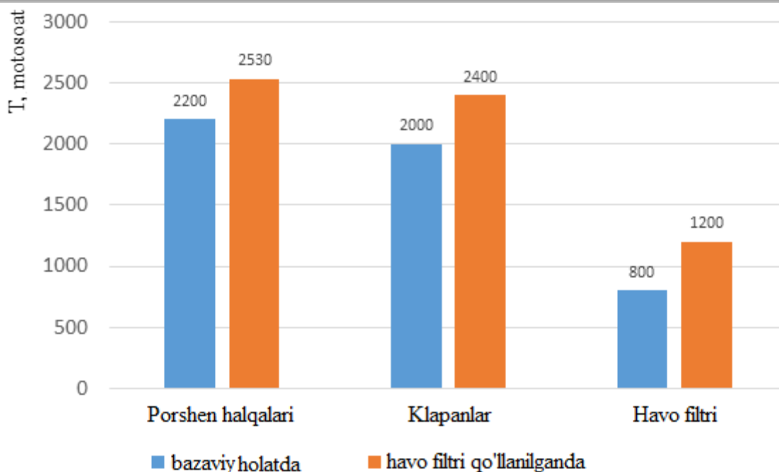
3-rasm. Kompessorga so‘riluvchi havoni tozalash filtrini qo‘llaganda va bazaviy holatda ishchi qismlarning ish resursi
