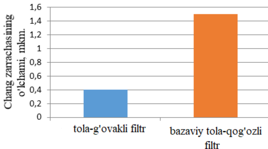
2-rasm. Tola-g'ovakli va tola-qog'ozli filtrni qo'llaganda filtrdan o'tgan havo tarkibidagi chang zarrachalarini o'rtacha o'lchami
