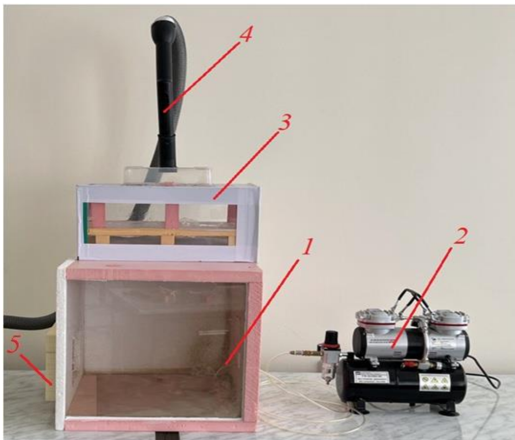
1 – sunʼiy chang hosil qilish kamerasi; 2 – kompressor; 3 – filtr; 4 – havo soʻrish quvuri; 5 – havo tuynigi
