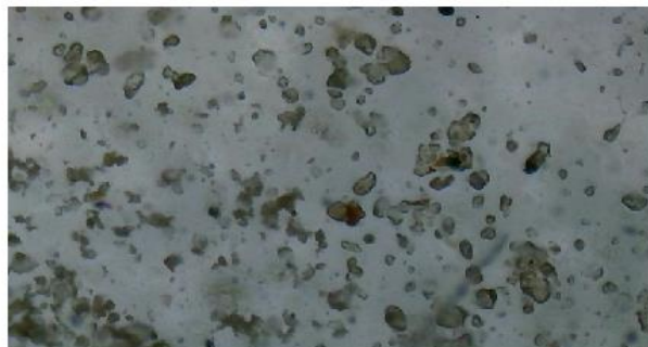
3-rasm. Ishlab chiqilgan (a) va bazaviy (b) filtrni qo'llaganda filtrdan o'tgan havo tarkibidagi chang zarrachalarini mikroskopik tasviri
