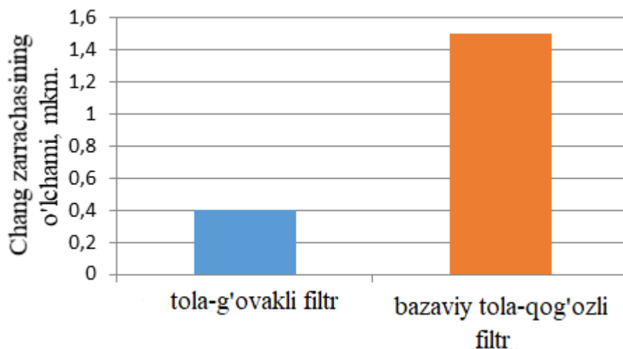
4-rasm. Tola-g'ovakli va tola-qog'ozli filtrni qo'llaganda filtrdan o'tgan havo tarkibidagi chang zarrachalarini o'rtacha o'lchami
