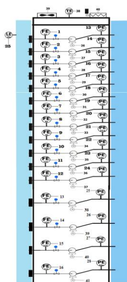
2-rasm Nasos stansiyasini avtomatlashtirish funksional sxemasi
