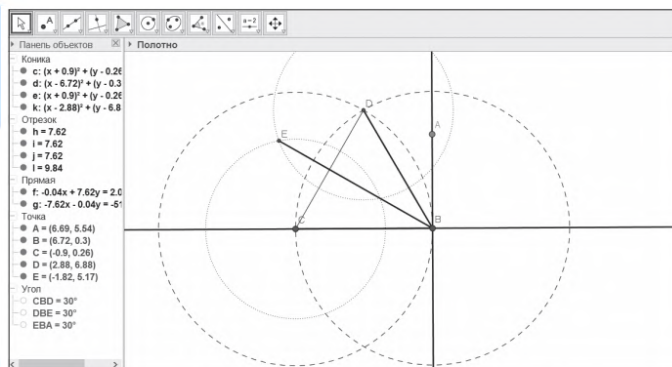
3-rasm. Al - Farabi algoritmi bo'yicha to'g'ri burchak triseksiyasini qurish
