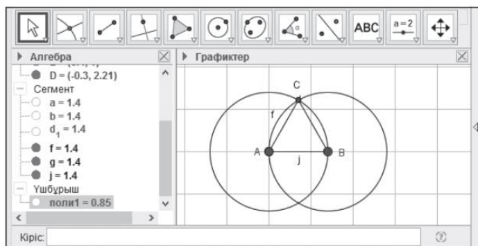
1-расм. Al - Farabi algoritmi bo'yicha teng tomonli uchburchakni qurish.
