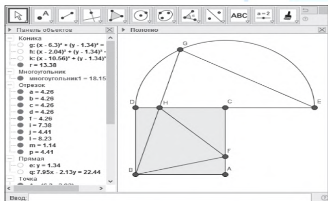
2-расм. Al - Farabi algoritmi bo'yicha kvadratga yozilgan teng tomonli uchburchakni qurish.
